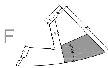
PLANTA NIVELL 179.70
