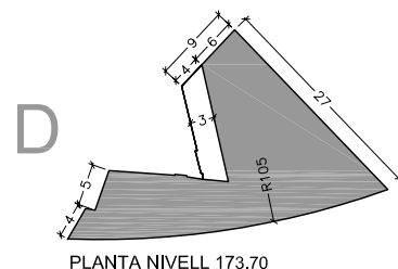
PLANTA NIVELL 173.70
