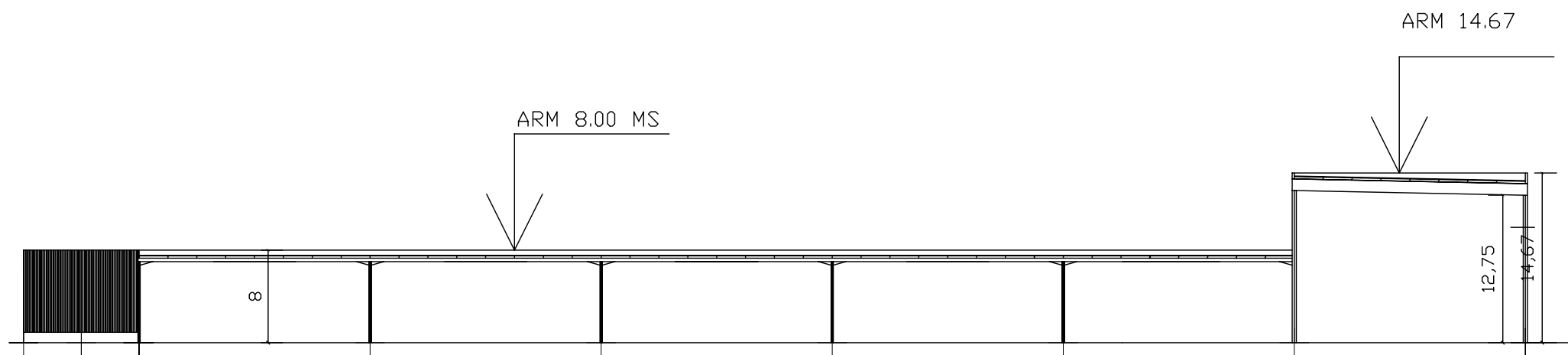
SECCIÓN A-A
