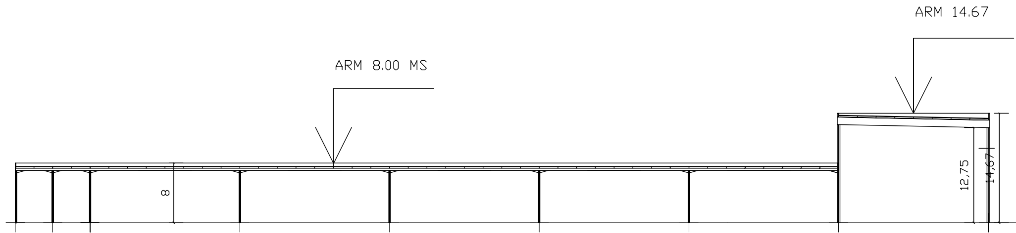
SECCIÓN B-B
